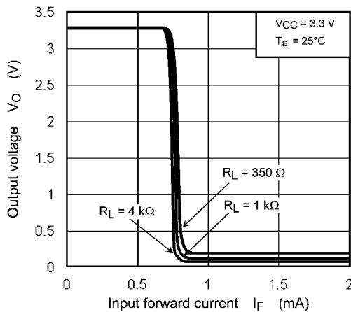
Fig. 12.2.6 V_O - I_F
