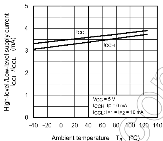
Fig. 12.2.9 I_{CCH}/I_{CCL} - T_a
