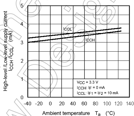
Fig. 12.2.10 I_{CCH}/I_{CCL} - T_a
