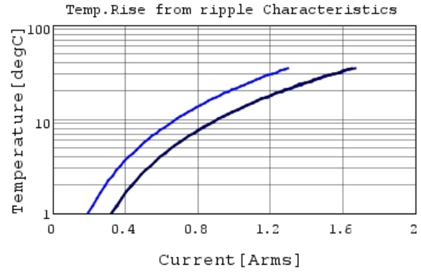
GRM188R72A104KA35 Temp.rise — 400kHz —
