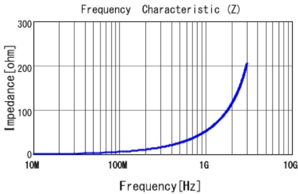
LQP03TN8N2H02 |Z|
