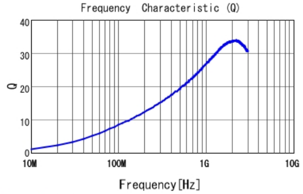
LQP03TN8N2H02 Q
