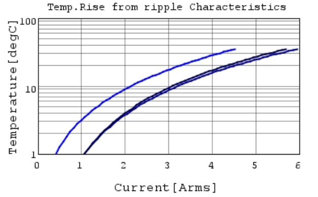
GCM31CR70J226ME23 Temp.rise — 80kHz
