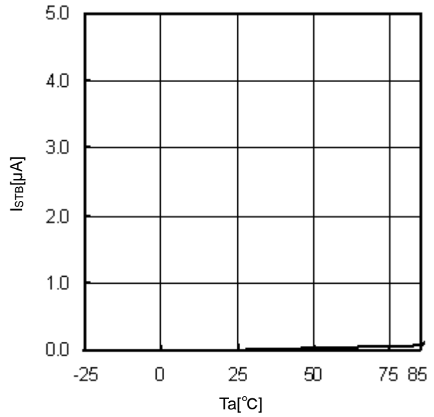
Fig.12 Ta-Istb (VEN=0V)
