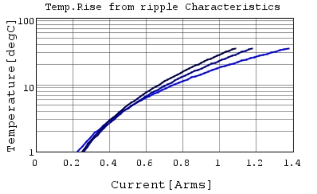
GRT1555C1H101JA02 Temp.rise — 200MHz
