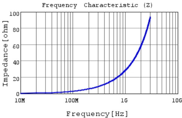
LQW15AN4N7C00 |Z|
