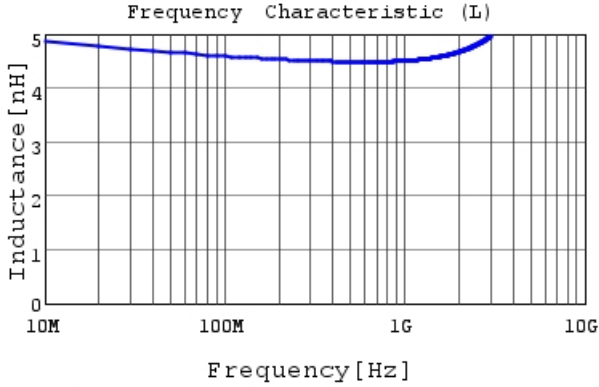
LQW15AN4N7C00 L
