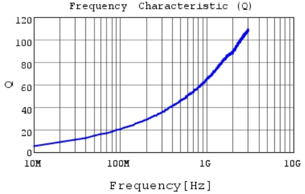
LQW15AN4N7C00 Q
