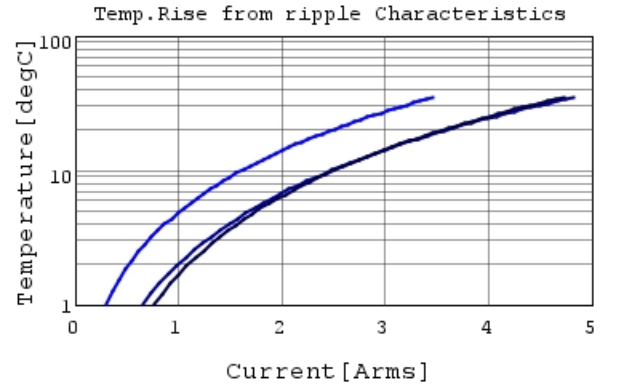
GRM319R6YA106KA12 Temp.rise — 80kHz —
