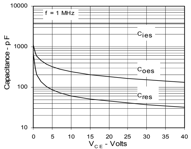
Fig. 12. Capacitance
