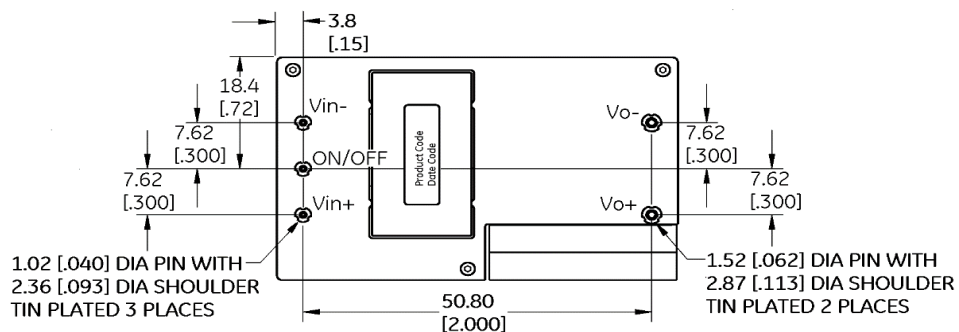
BOTTOM VIEW***
