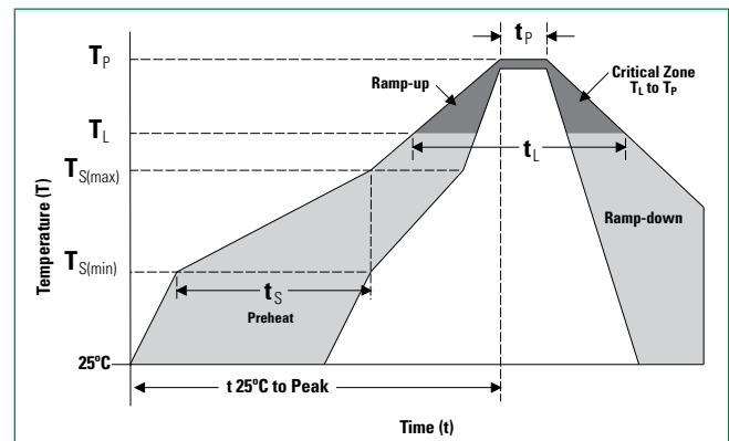
Soldering Parameters
