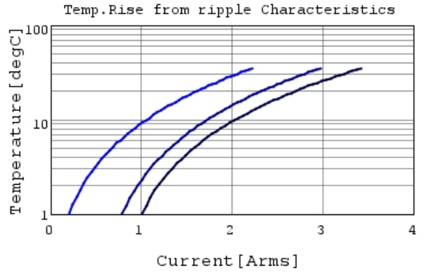
GRM155R61A105KE15 Temp.rise — 100kHz —
