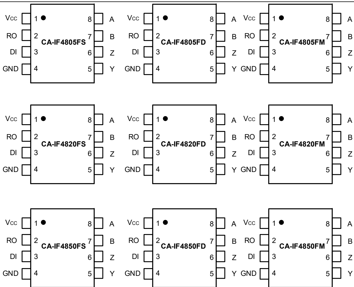
图 2 CA-IF48xxFS/CA-IF48xxFD/CA-IF48xxFM 引脚图
