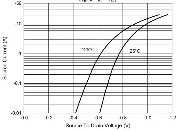
Fig. 9 - I_s - V_{SD}
