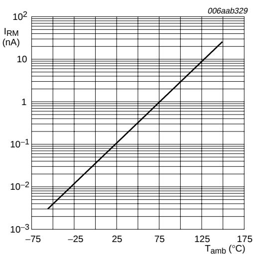
MMBZ27VCL: V_{RWM} = 22 \text{ V}
