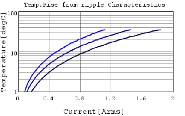
GRM155R71A474KE01 Temp.rise — 200kHz —
