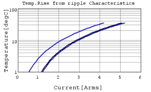
GRM185R60J106ME15 Temp.rise — 80kHz —
