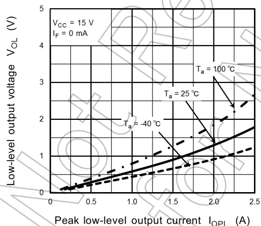
Fig. 13.2.11 V_{OL} - I_{OPL}
