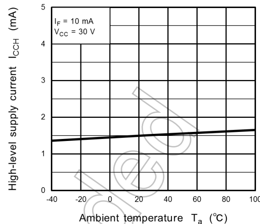
Fig. 13.2.8 I_{CCH} - T_a
