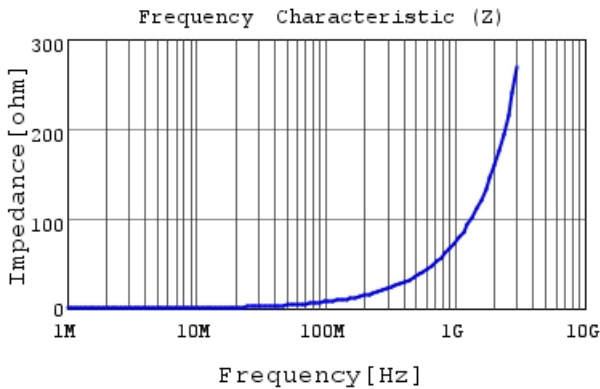
LQW15AN12NJ8Z |Z|
