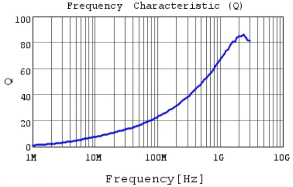
LQW15AN12NJ8Z Q
