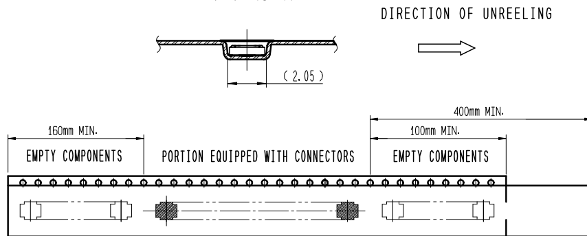
C-C (5:1)
