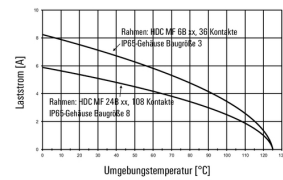
HDC-MHD 36-Module im IP65-Gehäuse, Leiter H07V-K2,5:
