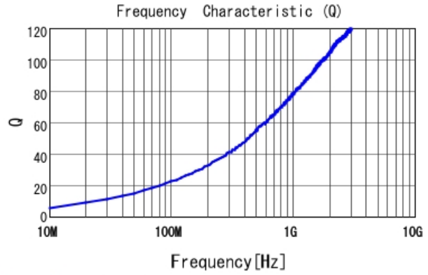
LQW15AN3N5C10 Q
