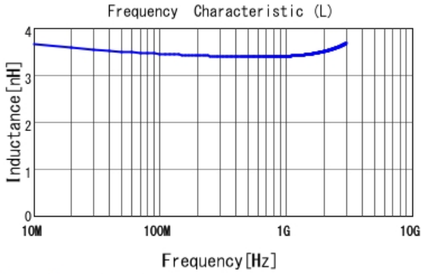
LQW15AN3N5C10 L
