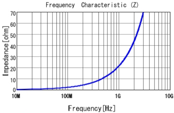
LQW15AN3N5C10 |Z|
