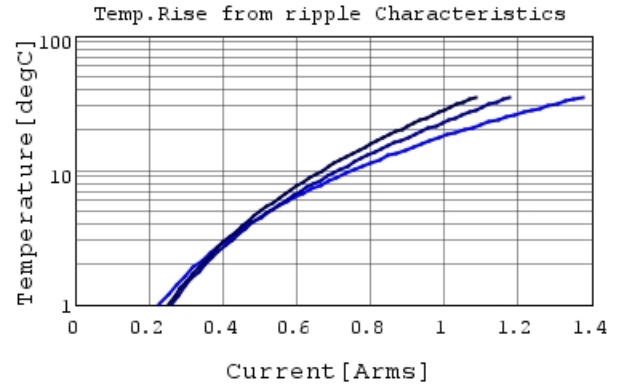
GRT1555C2A101JA02 Temp.rise — 200MHz
