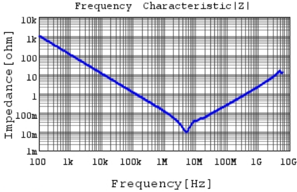
GCJ21BR71E225KA01 |Z| DCOV, 25degC
