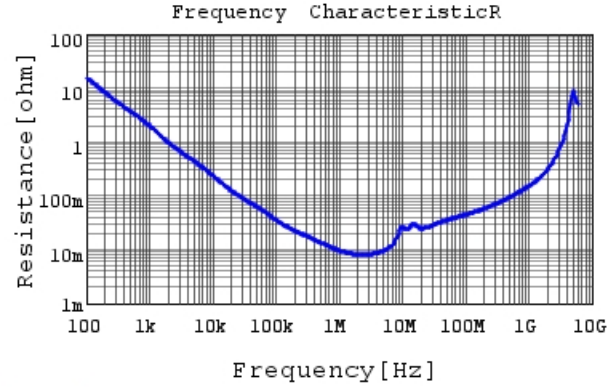
GCJ21BR71E225KA01 R DCOV, 25degC
