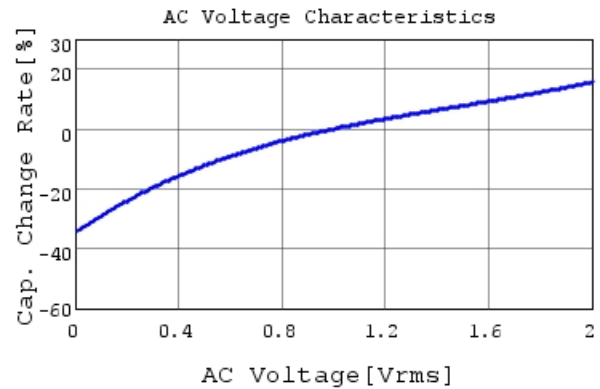
GCJ21BR71E225KA01 C-AC Voltage capchange, Dc
