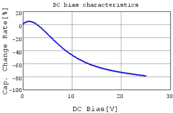
GCJ21BR71E225KA01 C-DC bias capchange, 25.0c
