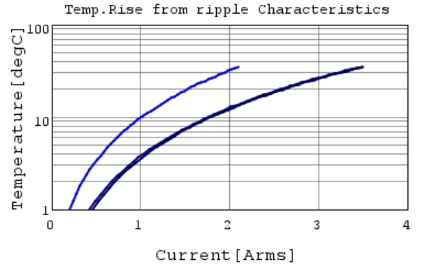
GCJ21BR71E225KA01 Temp.rise — 100kHz —
