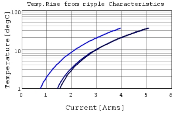
GRM155C80J106ME18 Temp.rise — 80kHz —
