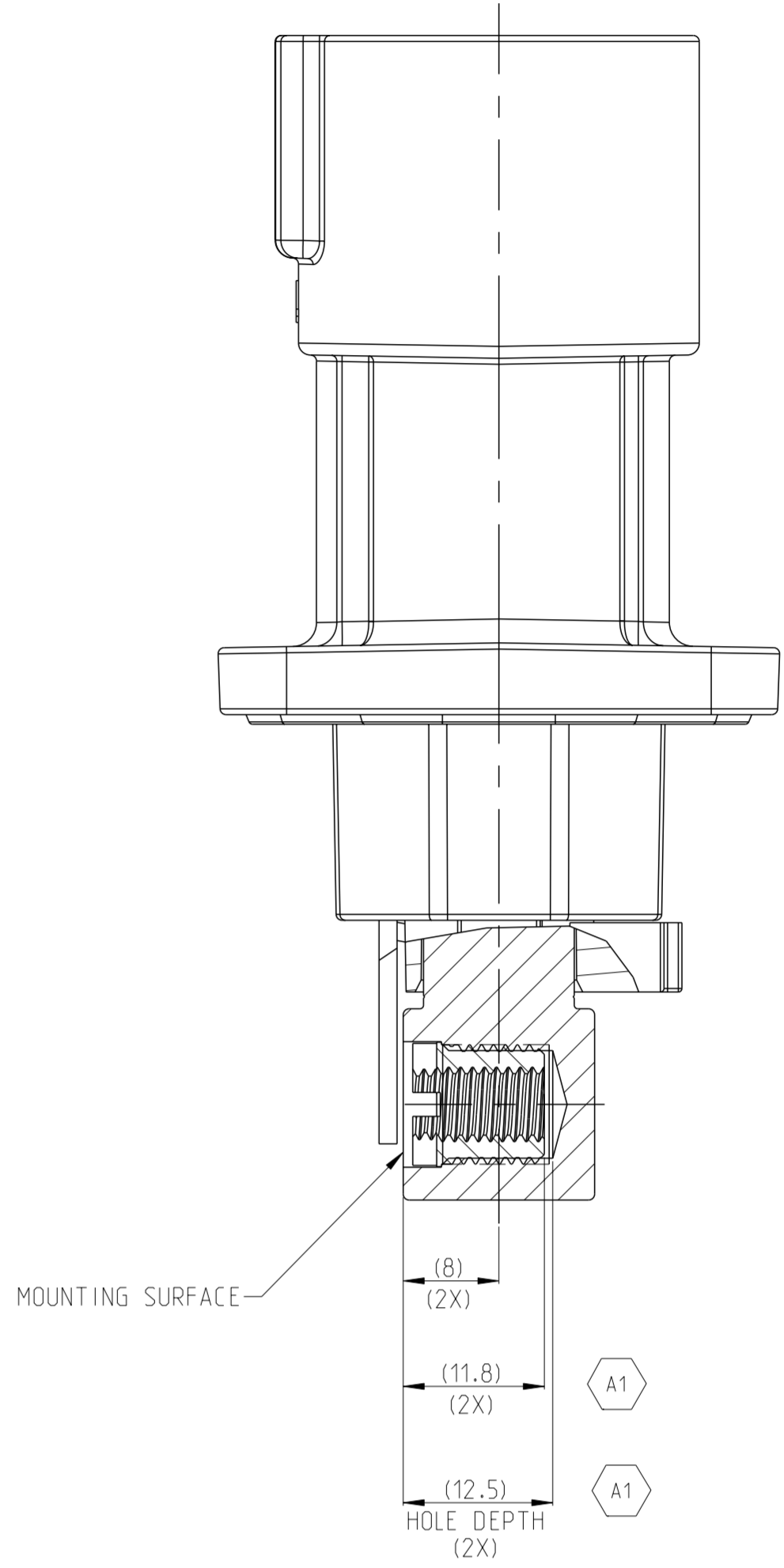
SECTION A-A
