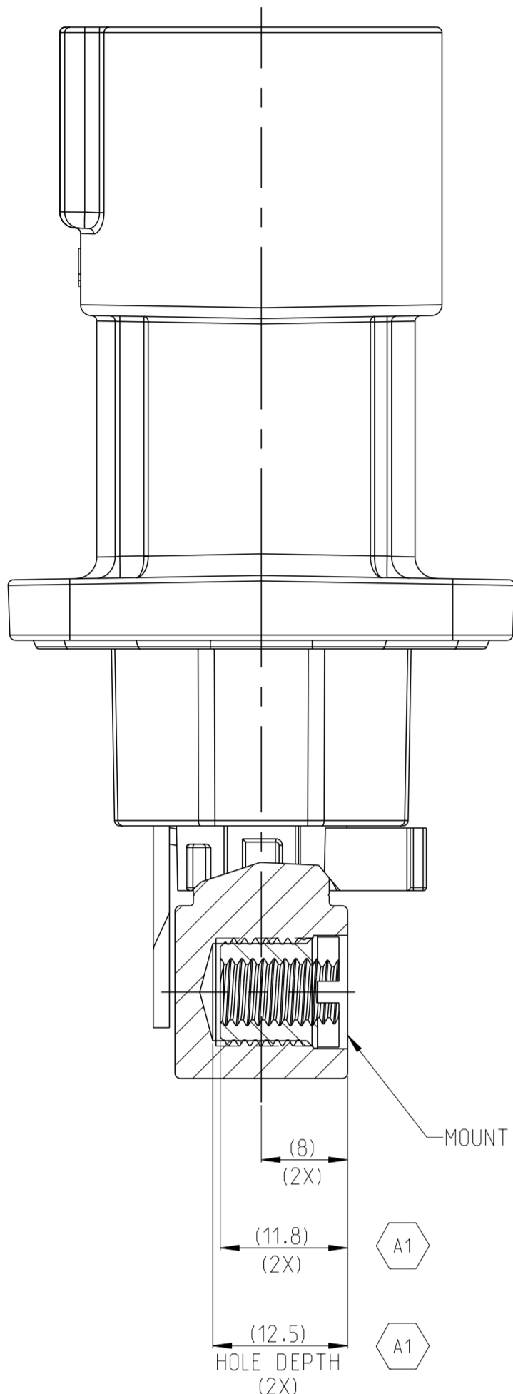
SECTION A-A
