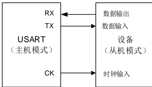
图 20-25. 同步模式下的 USART 示例
