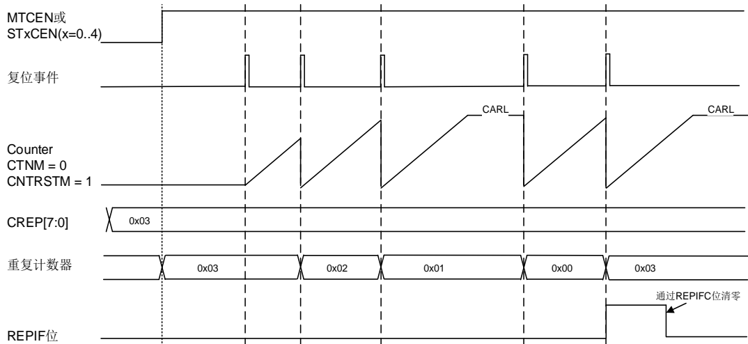
图 19-8. 单脉冲模式下，CNTSTM = 1 时重复计数器的动作
