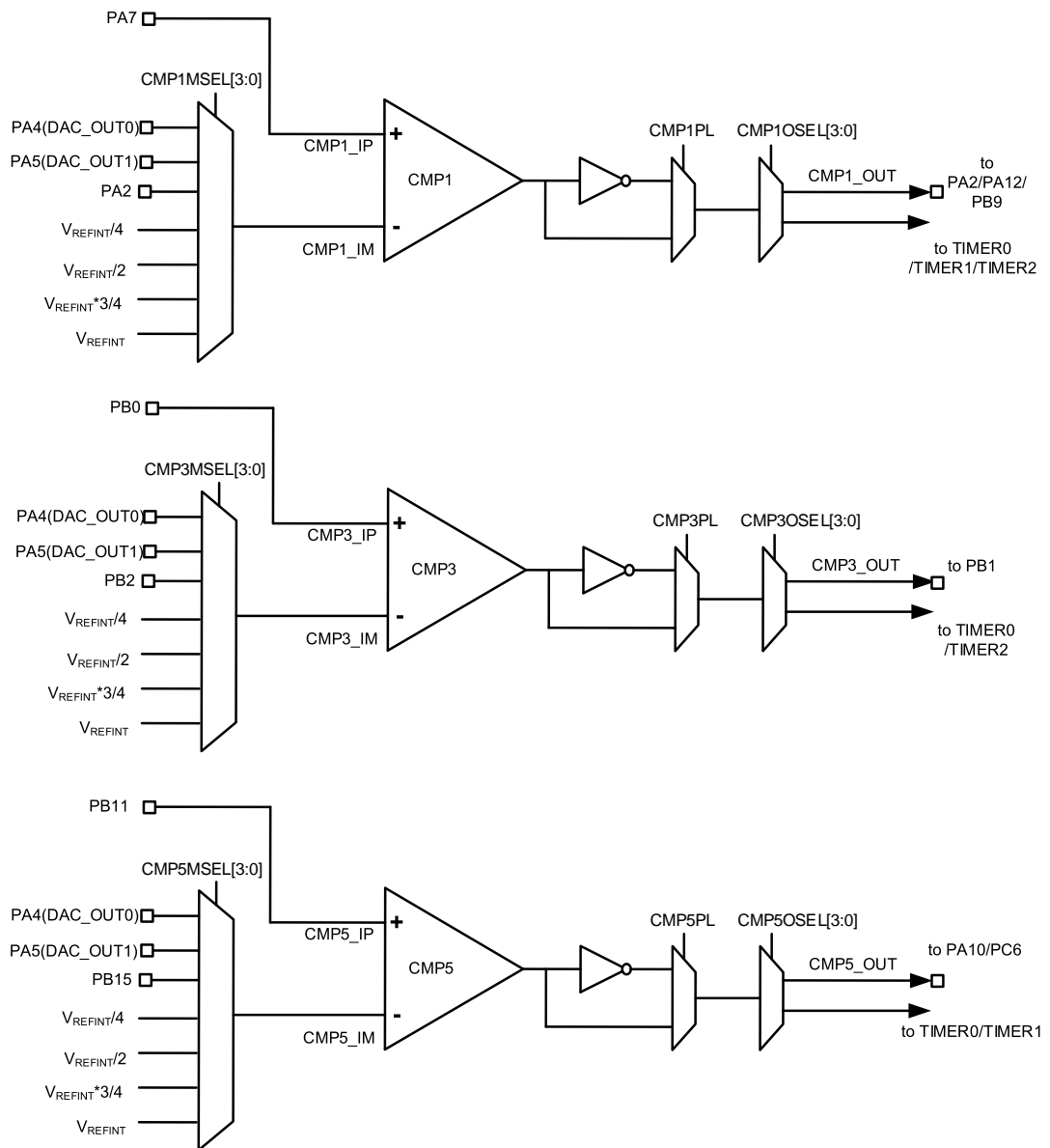
图 15-1. GD32E50x 芯片的比较器框图
