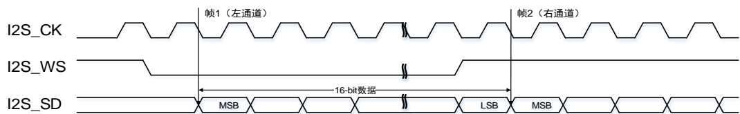
图 22-15. I2S 飞利浦标准时序图 (DTLEN=00, CHLEN=0, CKPL=0)
