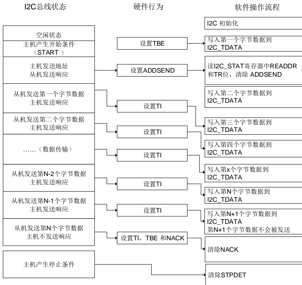
图 21-28. I2C 从机发送编程模型 (SS=1)
