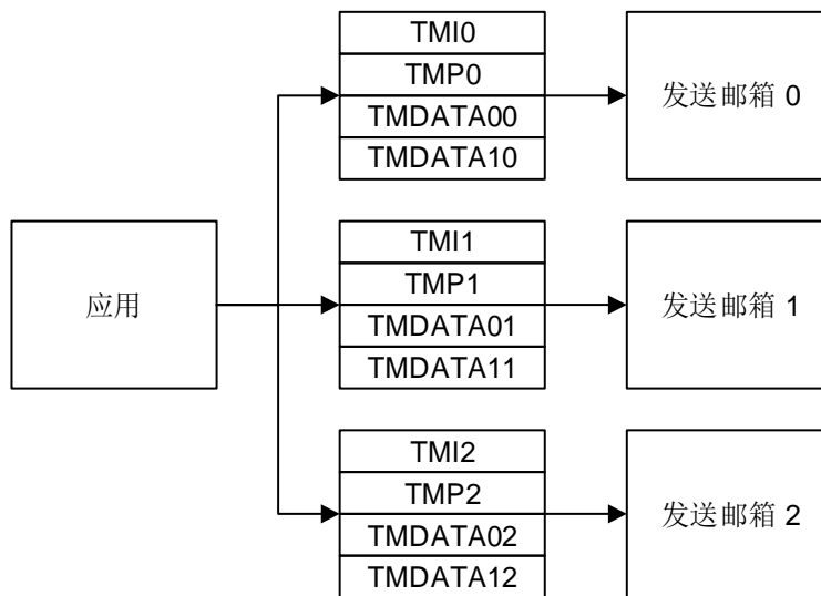
图 26-2. 发送寄存器
