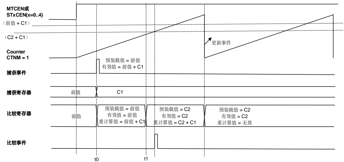
图 19-16. 比较延迟模式 (SHWEN=0)
