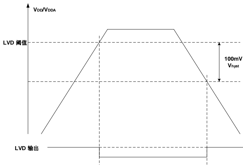
图 4-4. LVD 阈值波形图
