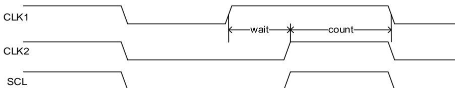
图 21-4. 时钟同步
