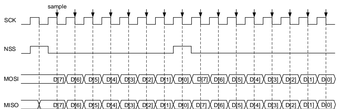
图 22-9. 主机 TI 模式在连续发送时的时序图
