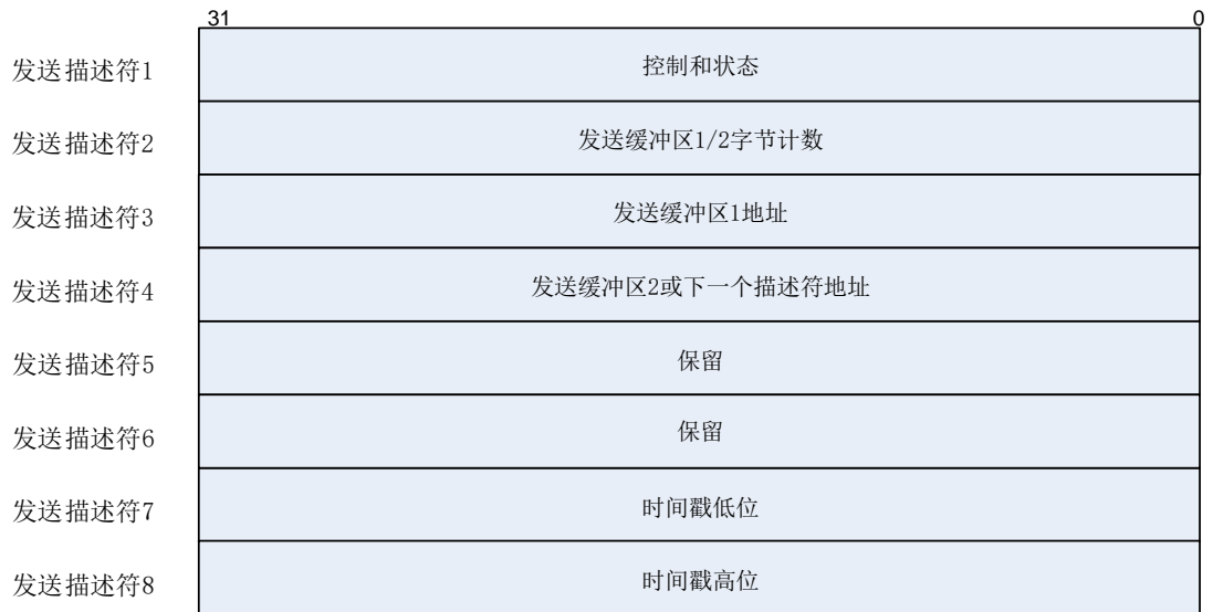
图 27-8. 增强发送描述符
