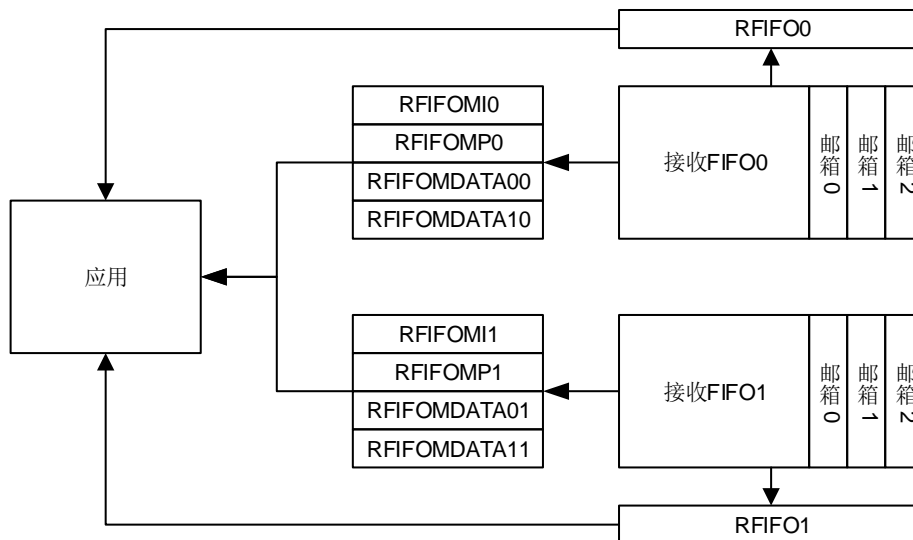
图 26-4. 接收寄存器
