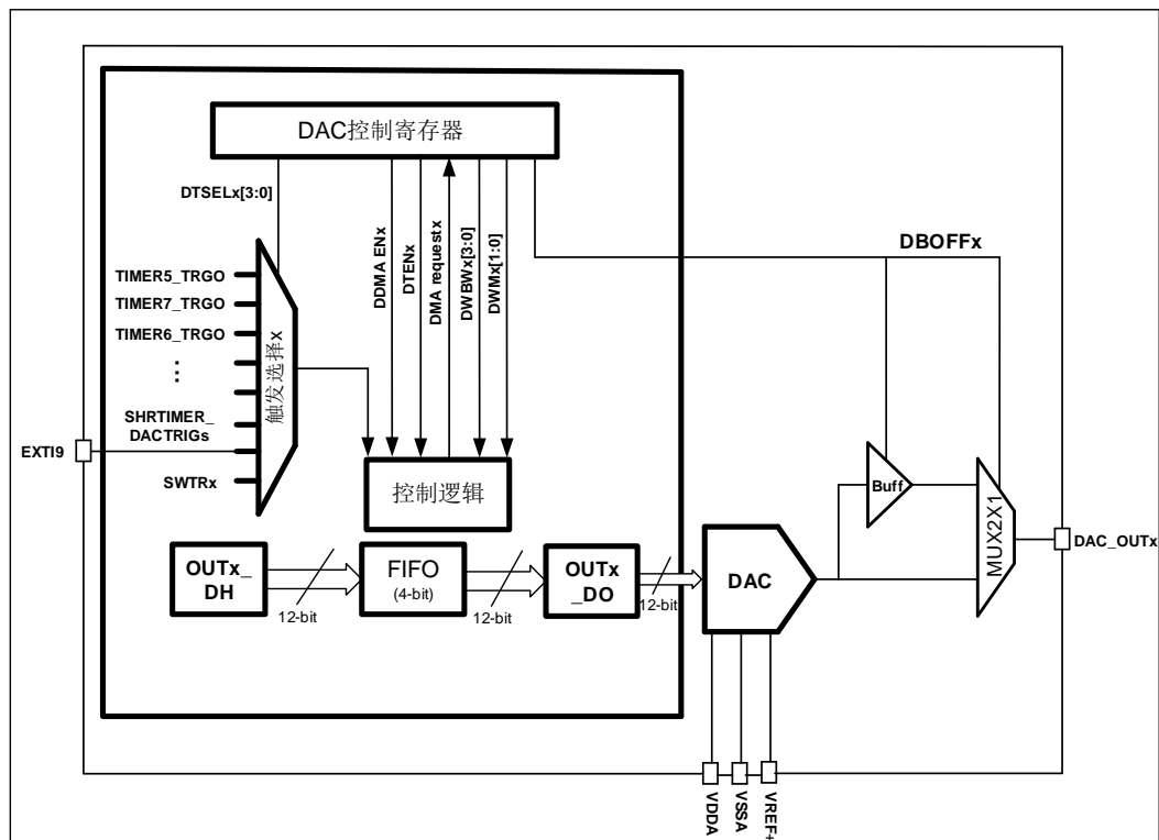
图 14-1. DAC 结构框图
