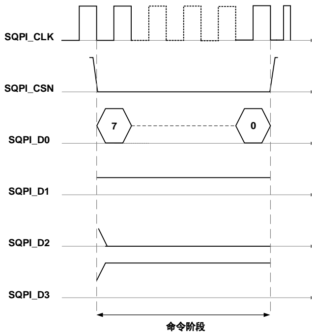
图 23-2. SQPI_SCMD 示例
