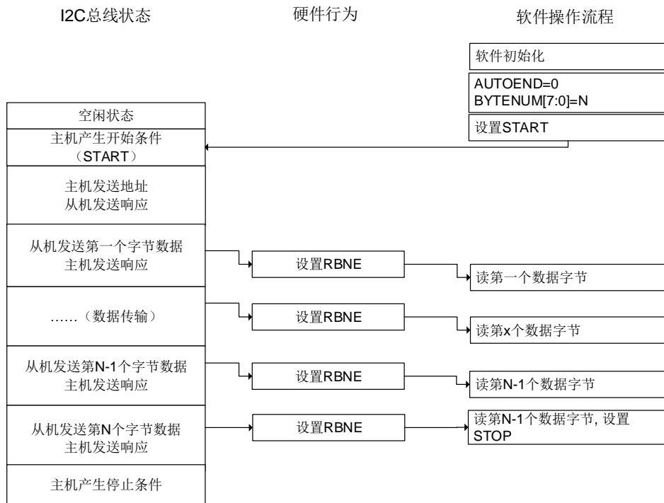
图 21-33. I2C 主机接收编程模型 (N<=255)
