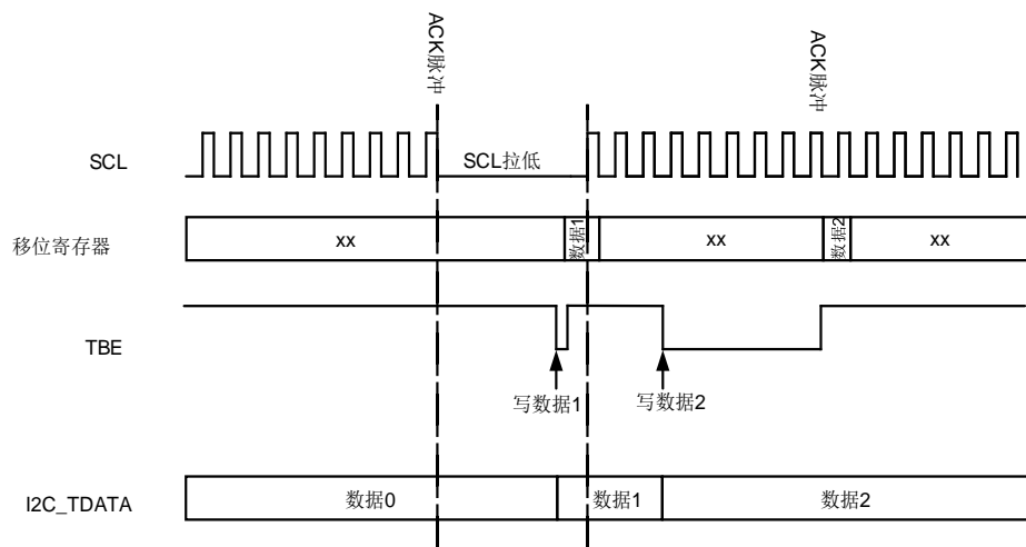
图 21-24. 数据发送
