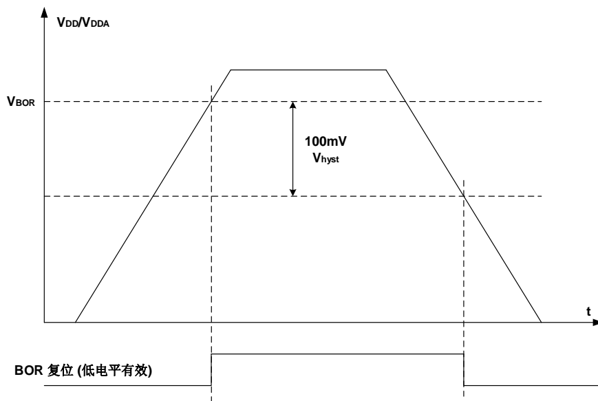
图4-3. BOR波形图
