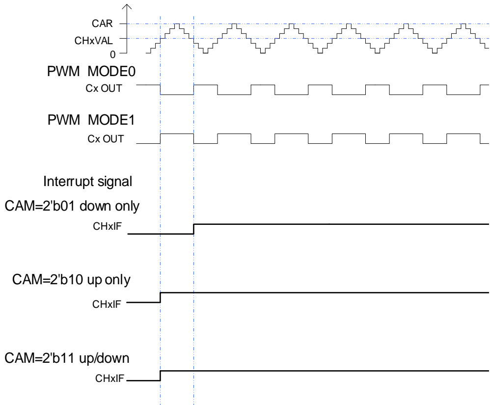
图 18-17. CAPWM 时序图
