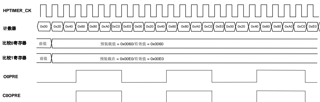
图 19-25. 常规模式下的 C0OPRE 波形
