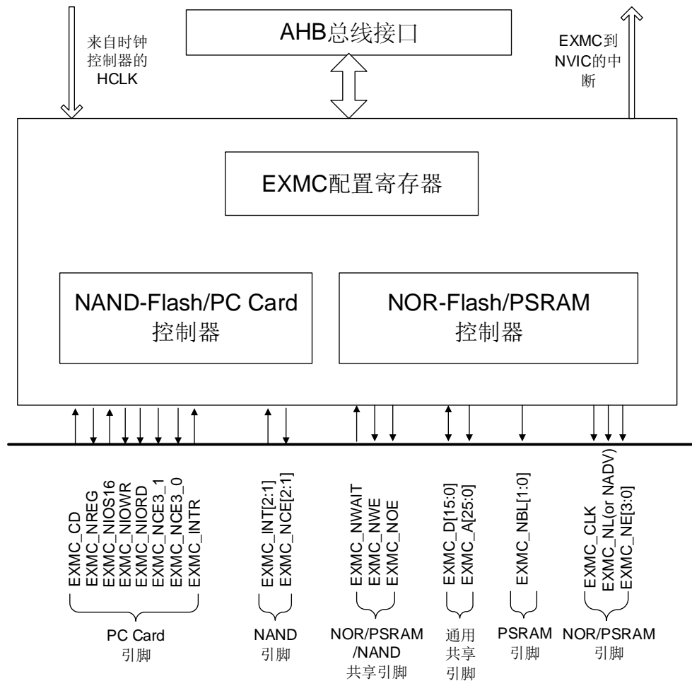
图 25-1. 系统架构
