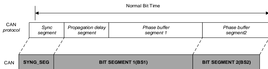
图 26-11. 位时序
