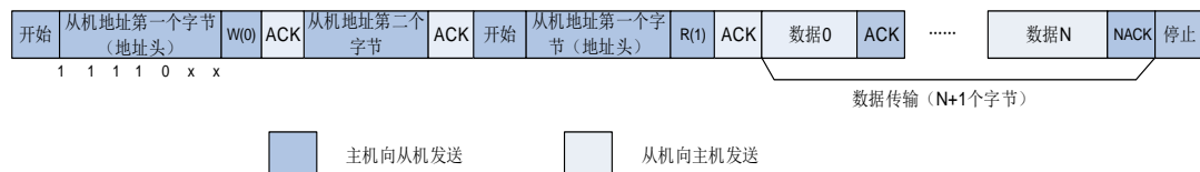
图 21-8. 10 位地址的 I2C 通讯流程（主机接收）
