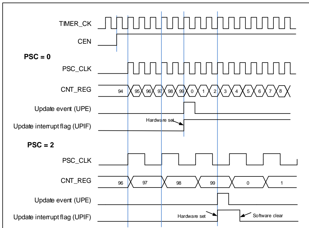
图 18-63. 向上计数时序图, PSC=0/2
