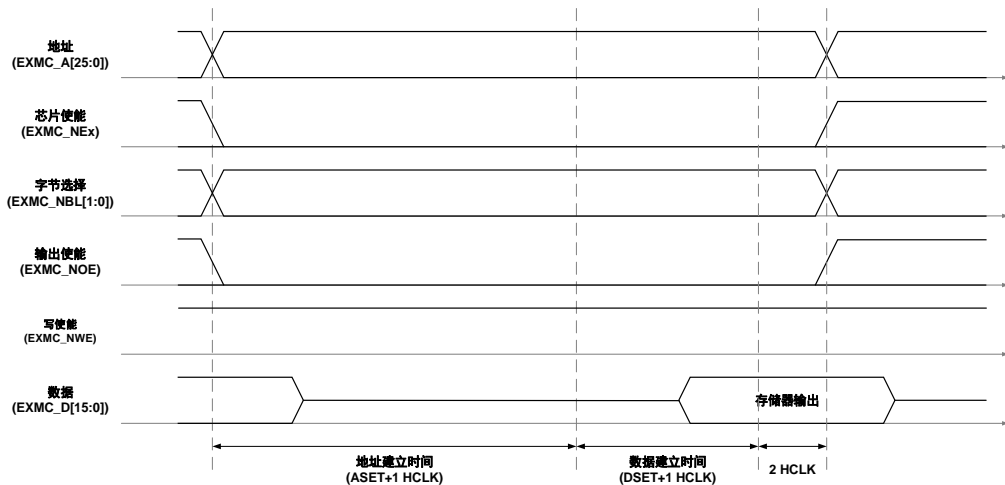
图 25-7. 模式 1 写时序
