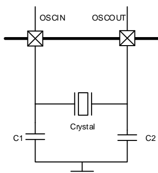
图5-3. HXTAL时钟源
