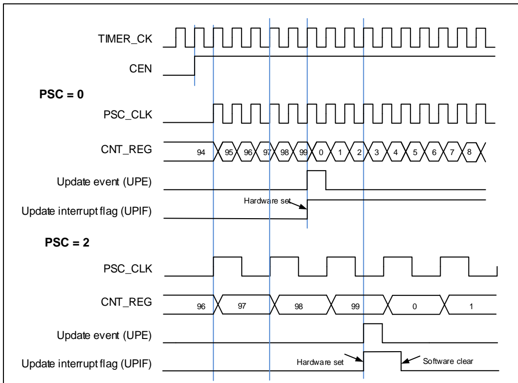
图 18-33. 向上计数时序图，PSC=0/2
