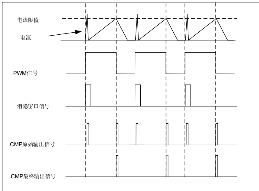
图 15-2. 比较器的输出消隐
