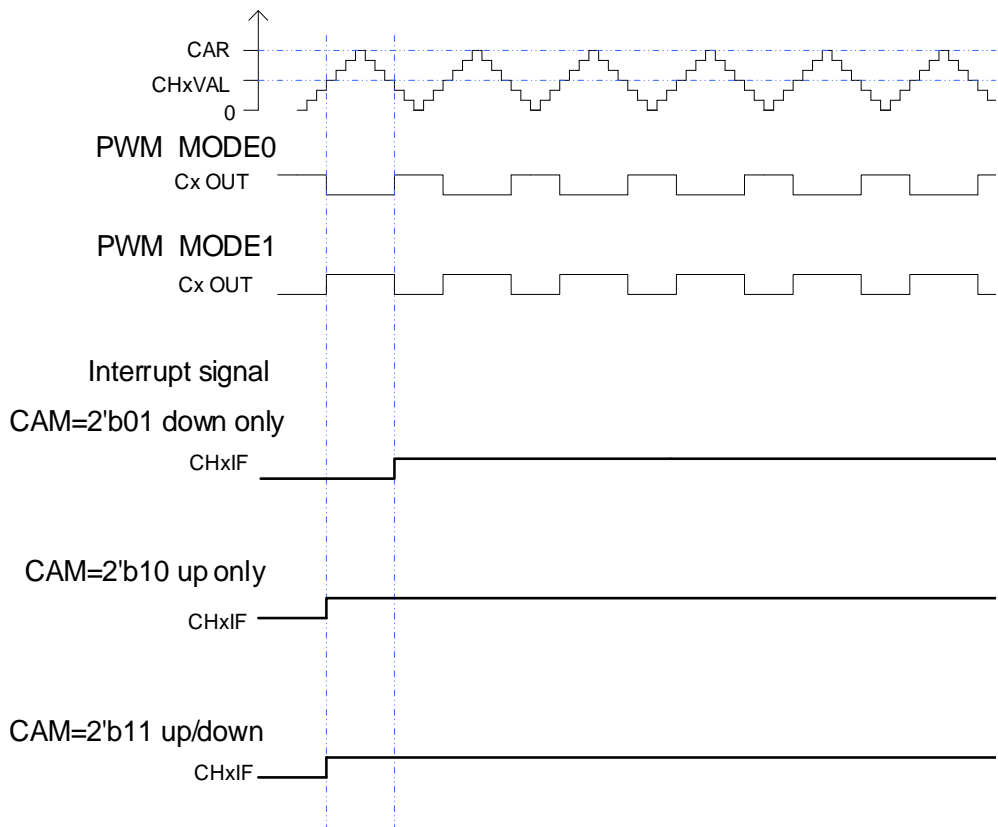
图 18-42. CAPWM 时序图
