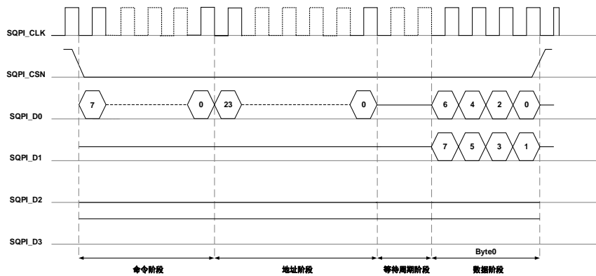
图 23-9. SQPI SSD 模式时序
