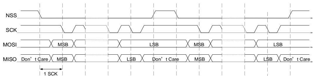
图 22-11. NSS 脉冲模式时序图（主机连续发送）
