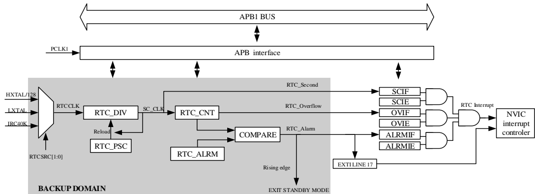
图 17-1. RTC 框图
