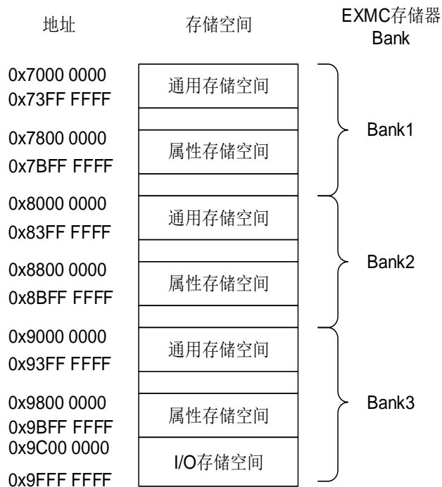
图 25-4. NAND/PC Card 地址映射
