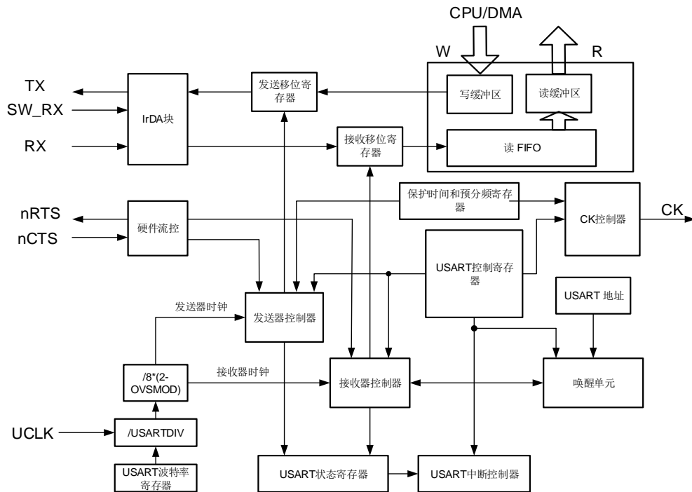
图 20-17. USART 模块内部框图
