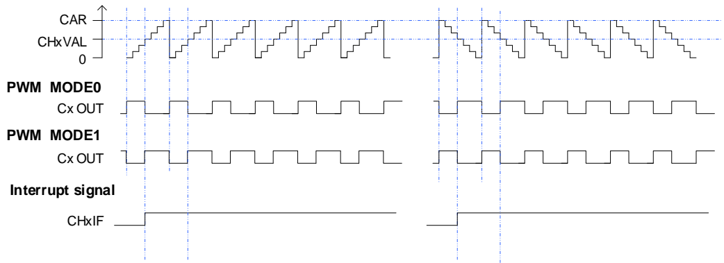
图 18-17. CAPWM 时序图
