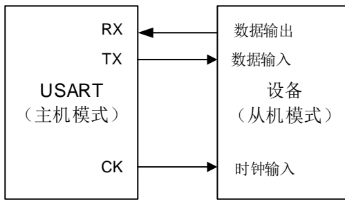
图 20-11. 同步模式下的 USART 示例
