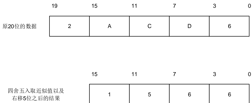
图 13-11. 右移 5 位和取整的教例
