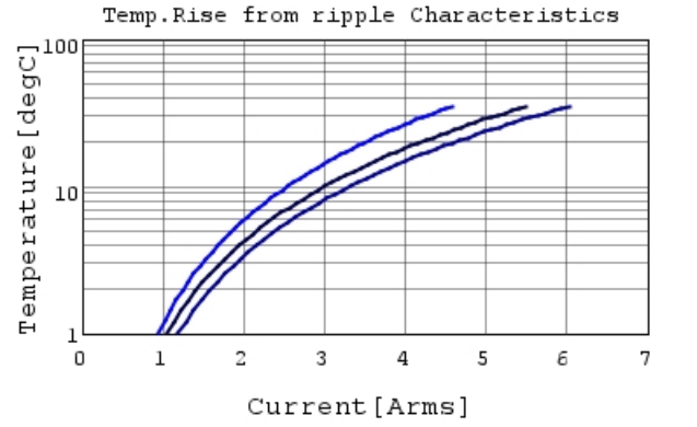
GRM32RR71C475KA01 Temp.rise — 100kHz —
