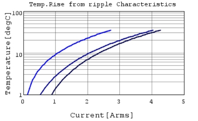
GRM21BR71A475KA73 Temp.rise — 100kHz —
