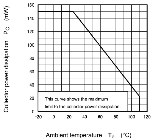
Fig. 11.2 P_C - T_a
